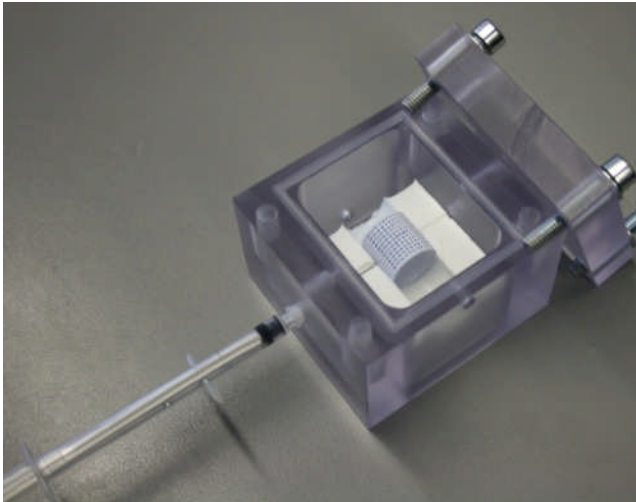
Miniatur-Nadelsensor: pH, O 2
